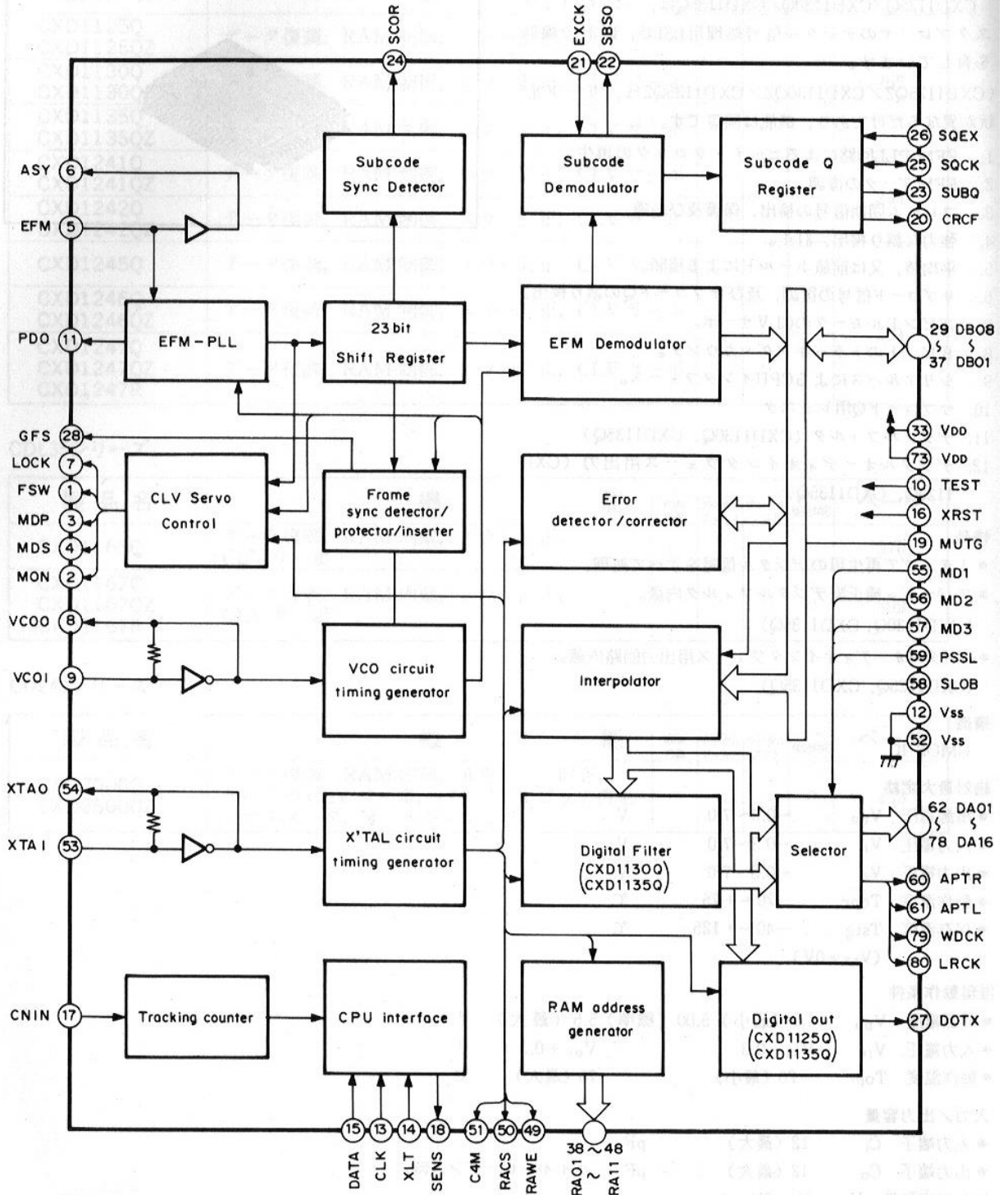
ブロック図
